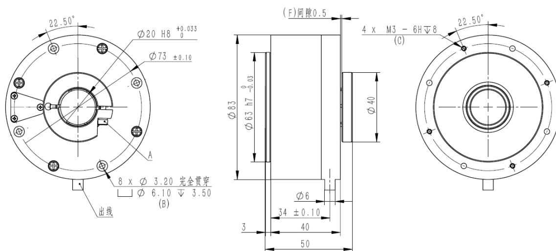
图1 外形尺寸图
