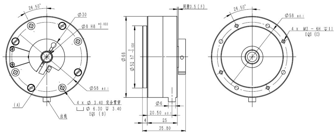
图1 外形尺寸图
